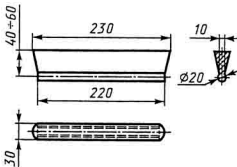
Рисунок 4 — Заготовка для вырезки образцов
