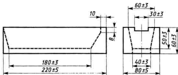
Рисунок 1 — Изложница
