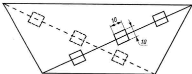
Рисунок Б.2 — Схема расположения квадратов на макрошлифе
